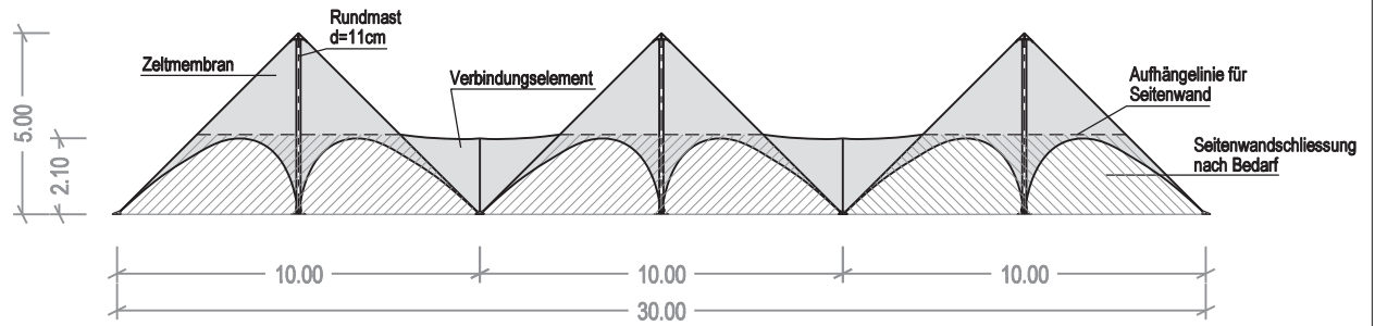
SCHNITT A-A
